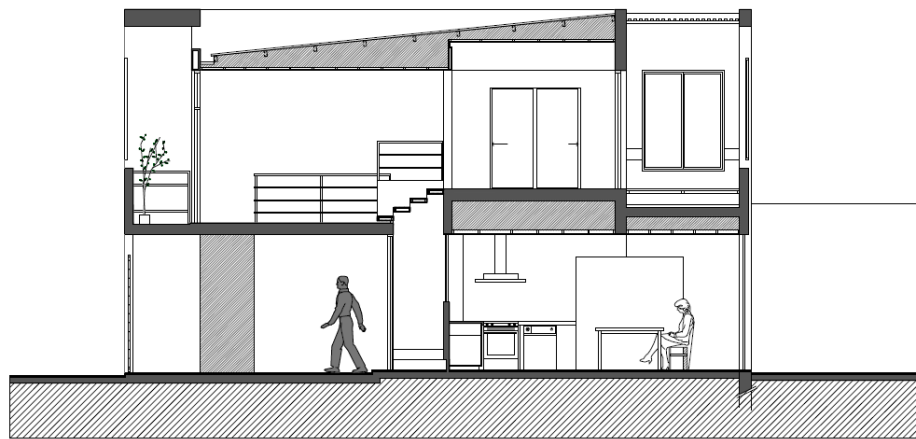
Corte Transversal
